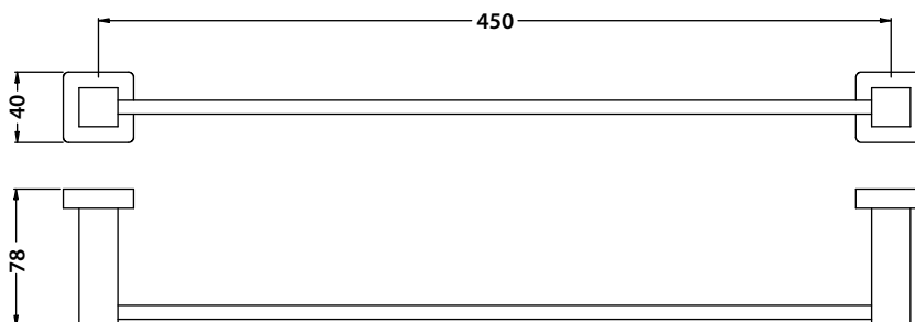
150.1009 Towel Bar - 18"
